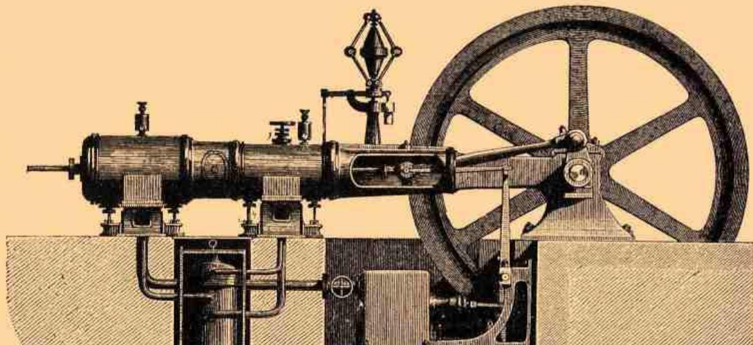
3. Горизонтальная паровая машина съ парораспределеніемъ Зульцера
