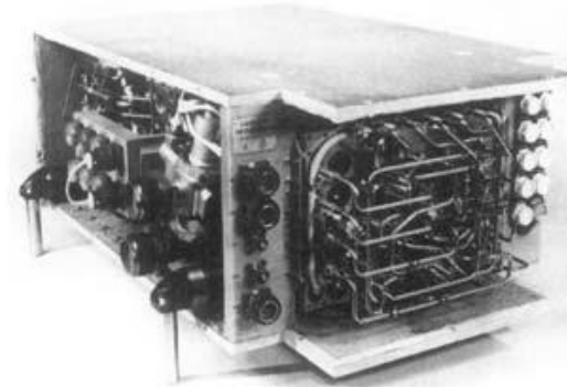
Батарея щелочных топливных элементов космического корабля «Буран» (СССР)
