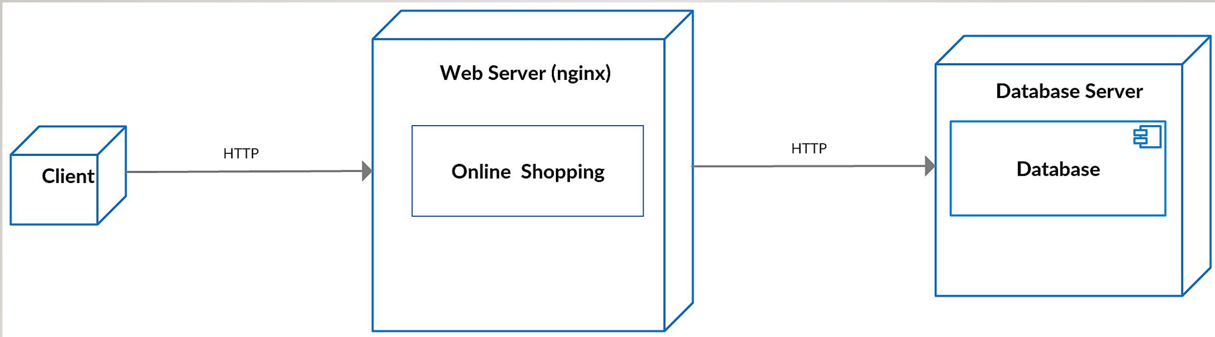
Рисунок 6 – Діаграма розгортання
