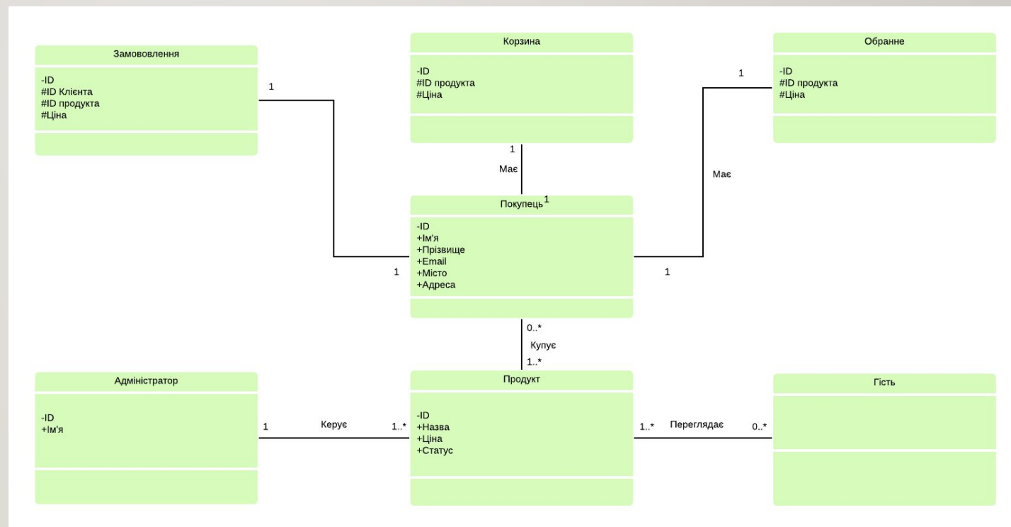
Рисунок 5 – Діаграма класів
