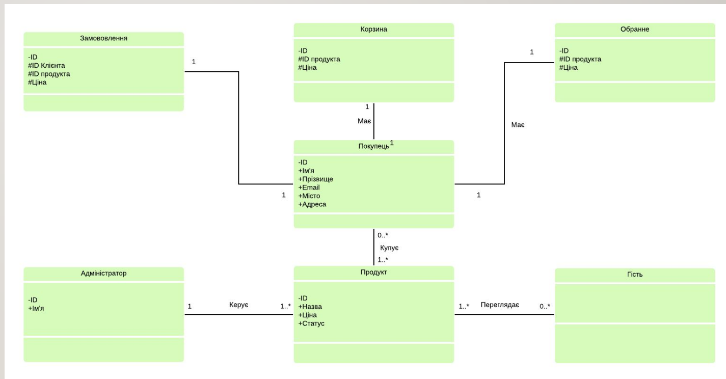
Рисунок 5 – Діаграма класів
