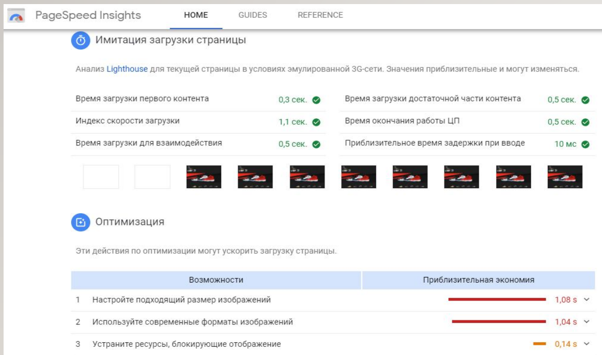
Рисунок 7 – Результат тесту на сервисі PageSpeed Insights
