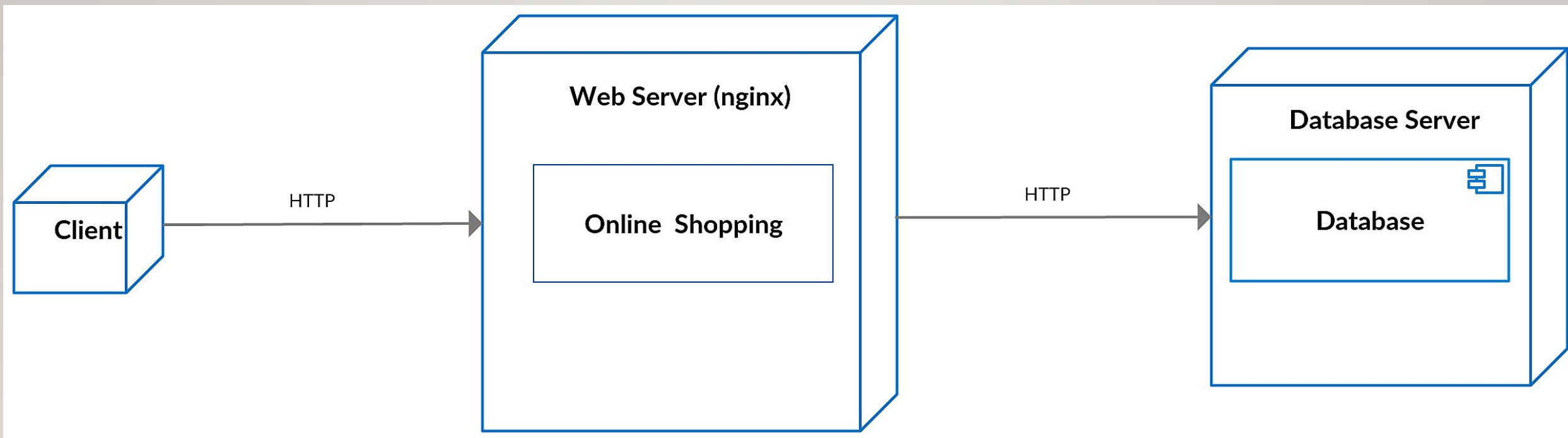
Рисунок 6 – Діаграма розгортання
