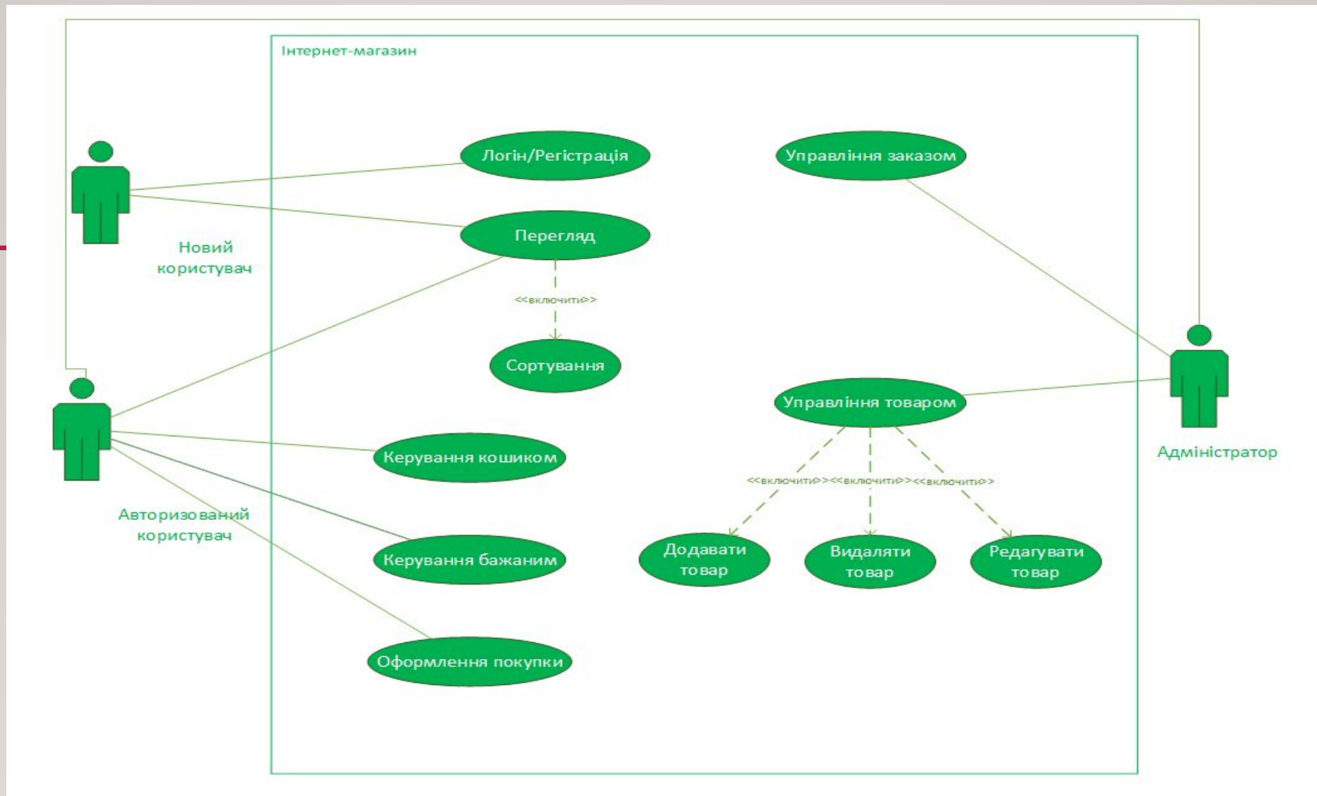
РИСУНОК 4 - ДІАГРАМА ПРЕЦЕДЕНТІВ
