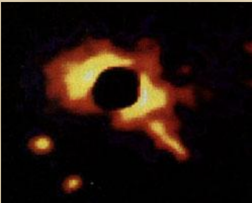
Самый ближний к нам квазар Маркарян 231 (3C 273), открытый в 1998г в 500 млн. св.лет от нас - центр эллиптической галактики (закрыт). Его возраст 1 млн. лет и проявляет себя как компактный радиоисточник. Через несколько миллионов лет его излучение раздует окружающее газообразное вещество и яркость квазара резко возрастет.
