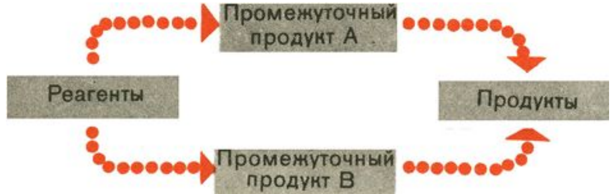
Схема цикла, иллюстрирующего закон Гесса
