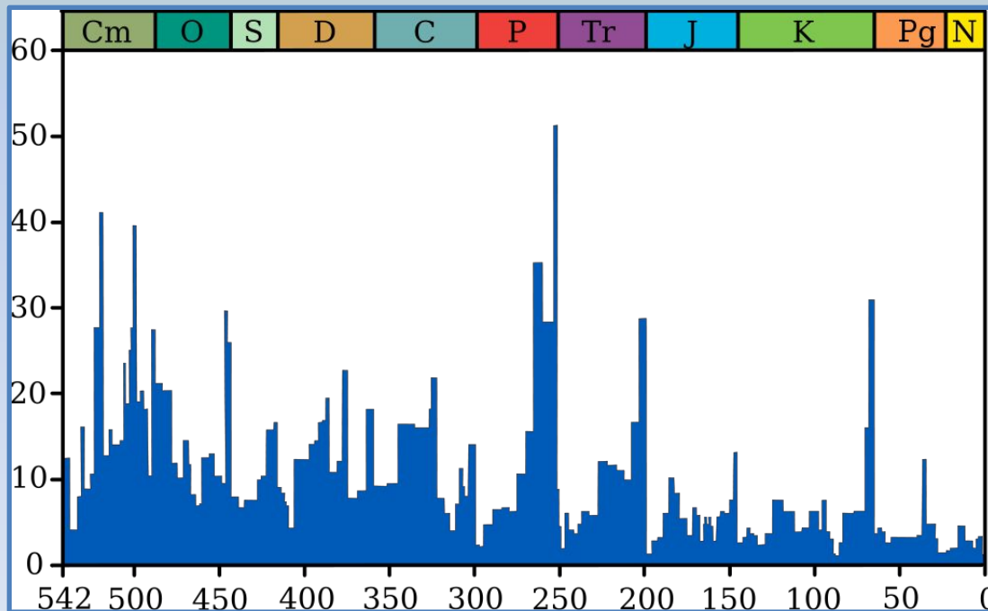
Вымирание морской фауны в фанерозое
