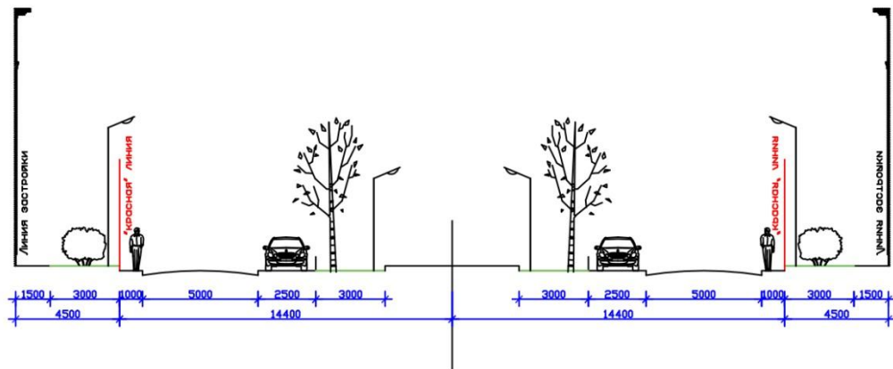
Профиль А-А Улица между домами №5-№6
