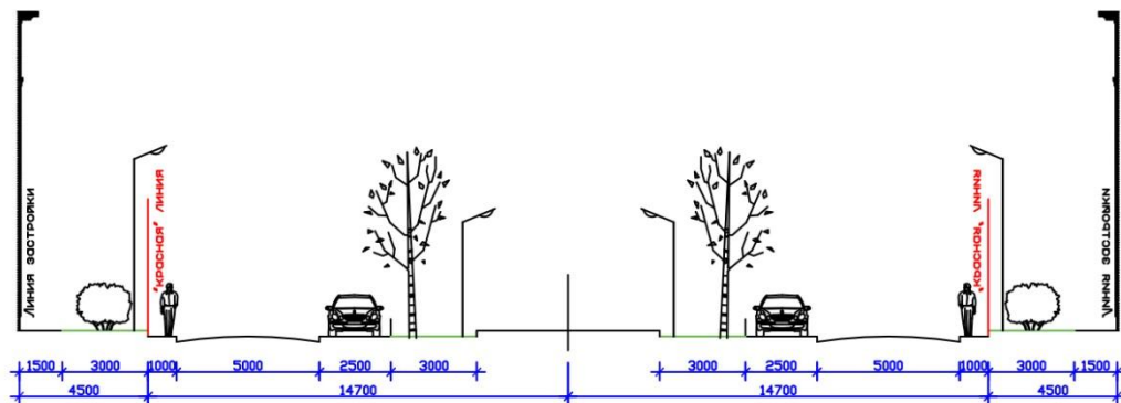
Профиль А-А Улица между домами №5-№7
