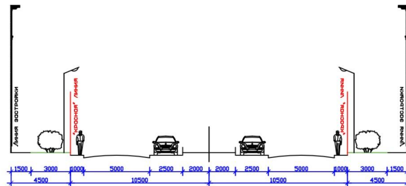
Профиль А-А Улица между домами №6-№7
