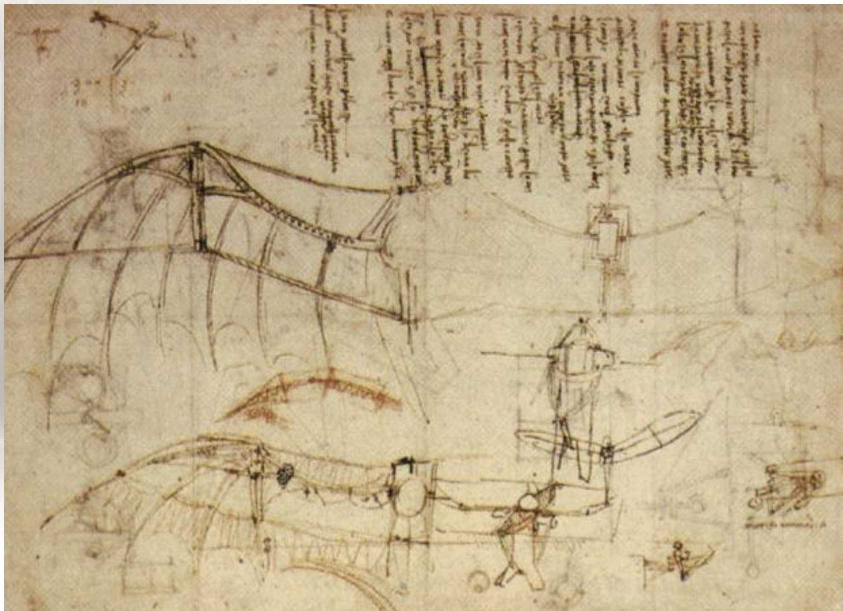
оригинальные чертежи
