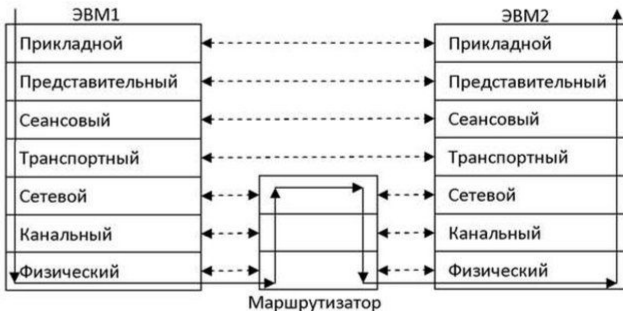
Рисунок – Взаимодействие двух ЭВМ в рамках модели OSI
