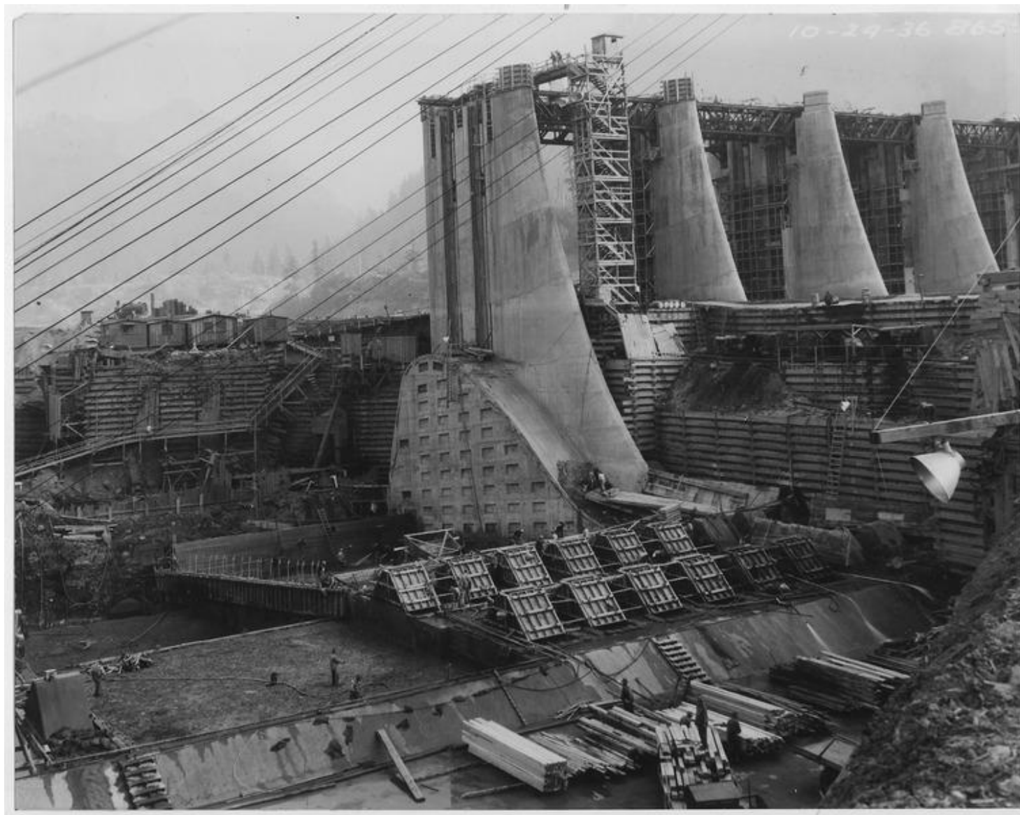
Сооружение плотины Бонневиль (штат Орегон), 1934-1937 гг.
