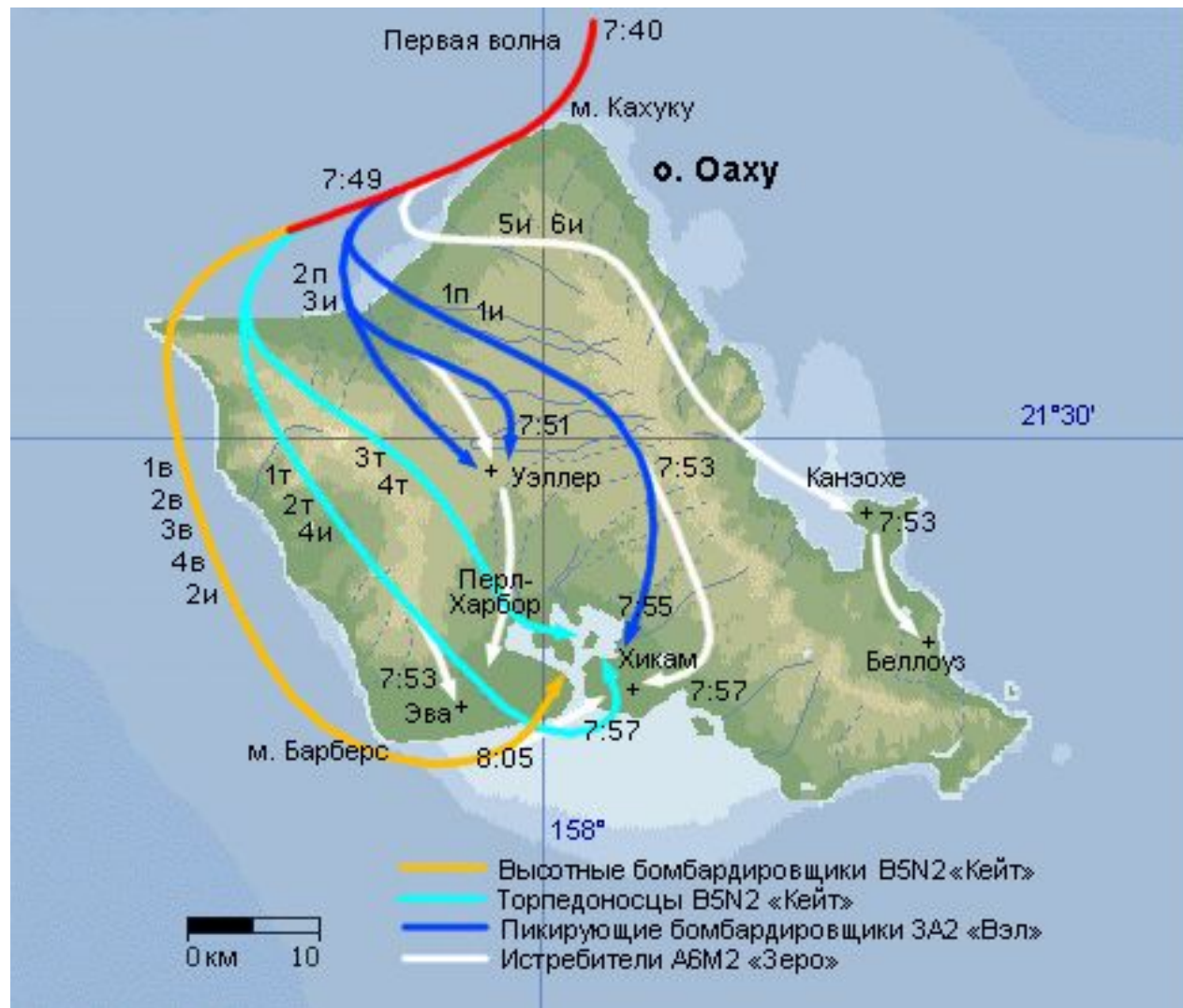
Схема первой волны японского авиаудара по базе Пёрл-Харбор, О. Оаху, Гавайские острова
