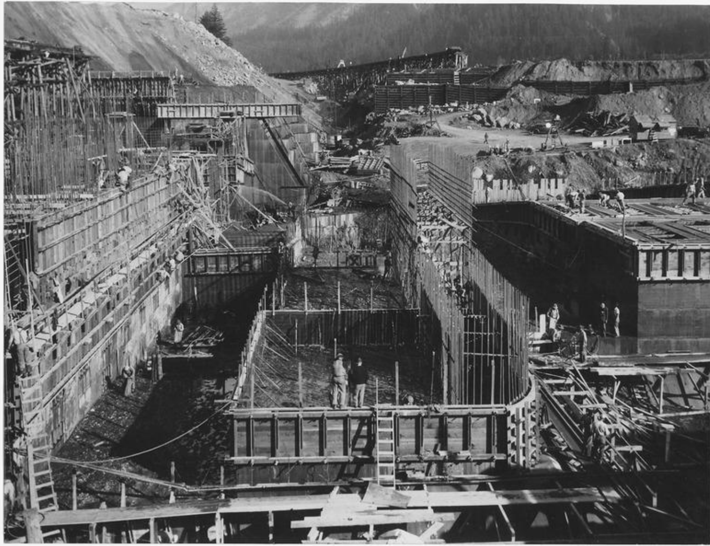
Сооружение плотины Бонневиль (штат Орегон), 1934-1937 гг.
