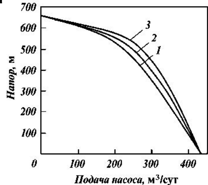
Рис. 3.18. График влияния свободного газа на рабочую характеристику насоса "Рэда" с центробежным газосепаратором при содержании газа на приеме насоса, \text{нм}^3/\text{м}^3 : 1 - 0; 2 - 0,20; 3 - 0,60.
