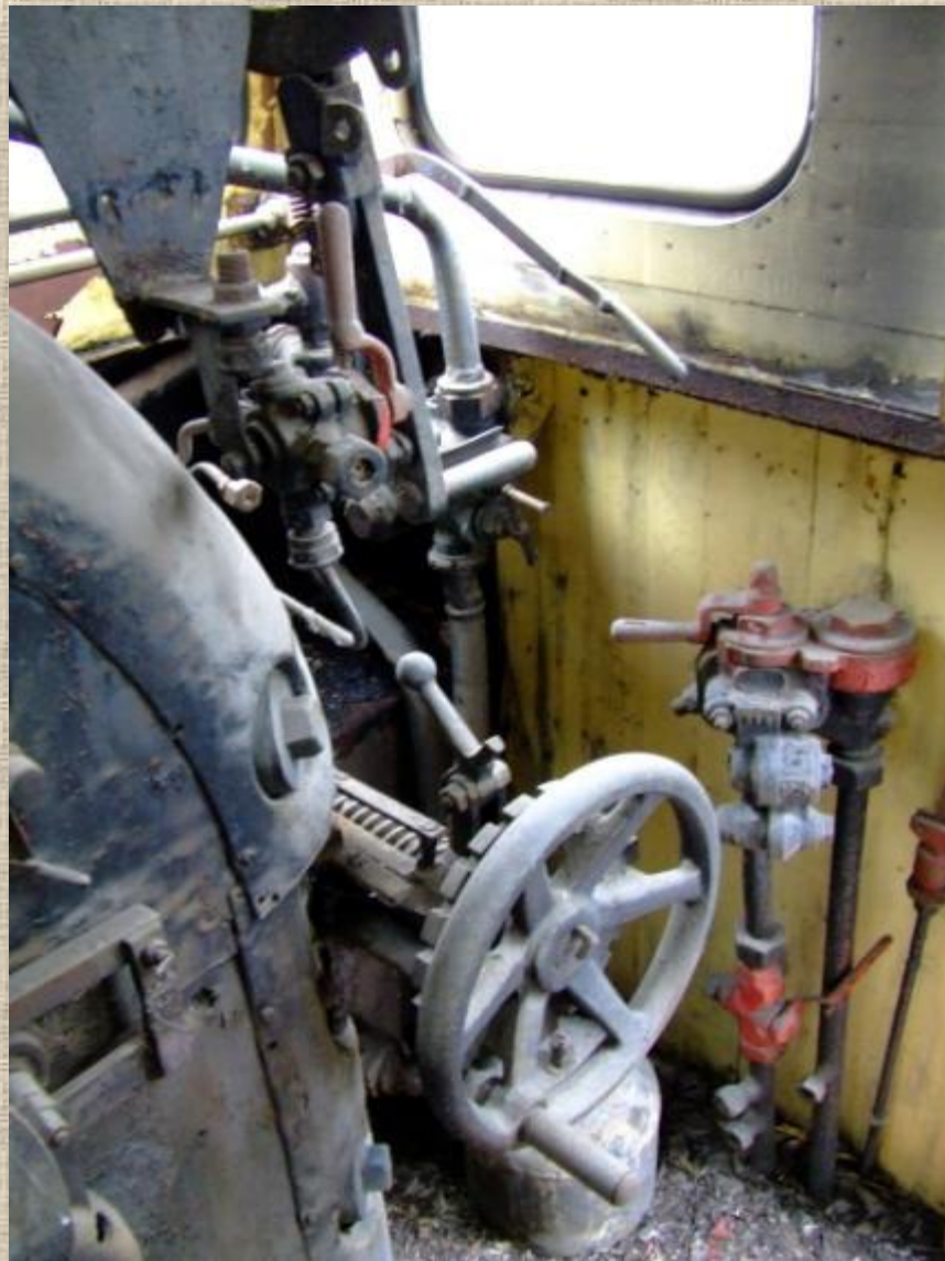
Кабина паровоза
