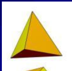
Тетраэдр
