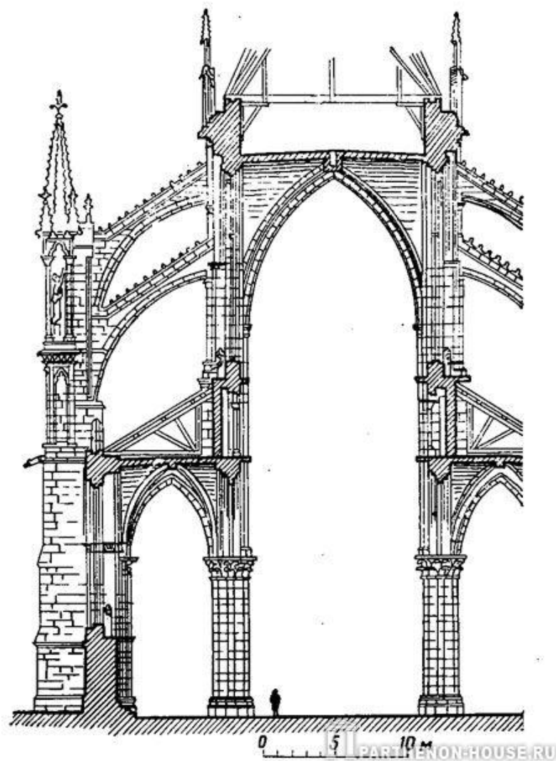
Каркасная система готической архитектуры
