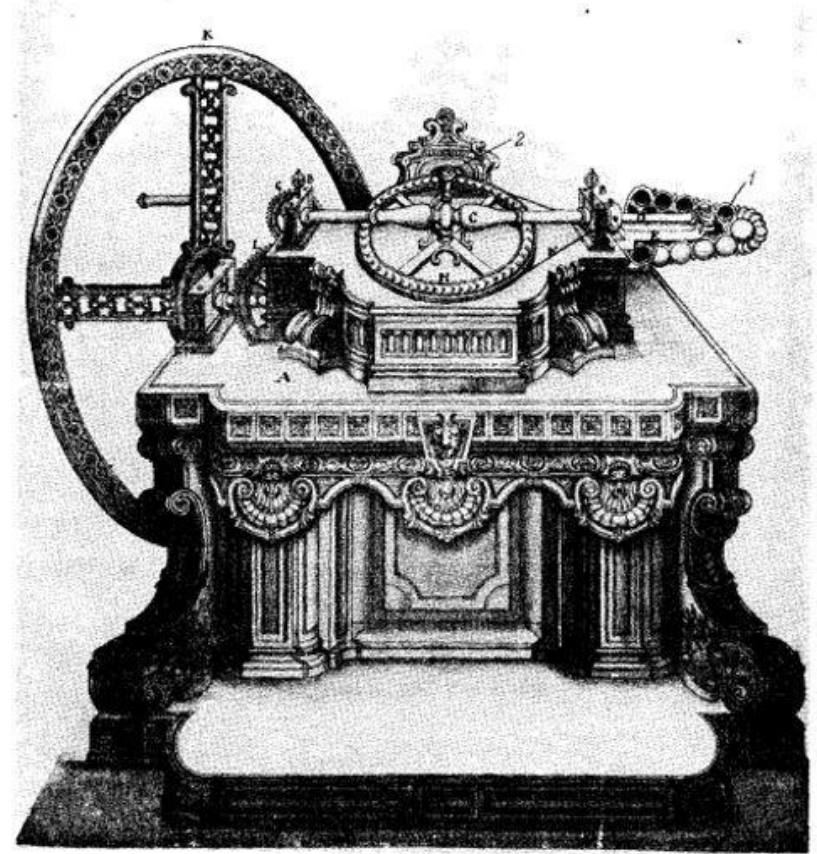
Рис. 113. Станок для фрезерования грибовидной фрезой. Рукопись «Театрум Махинарум» А. К. Нартова.
