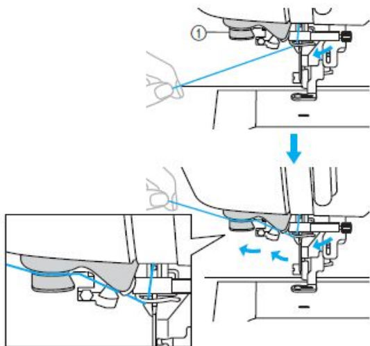
① Направляющий диск
