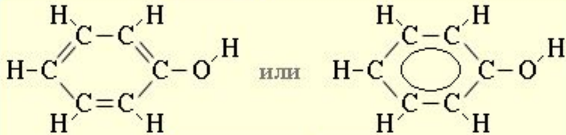
Структурные формулы
