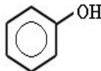
Фенол
