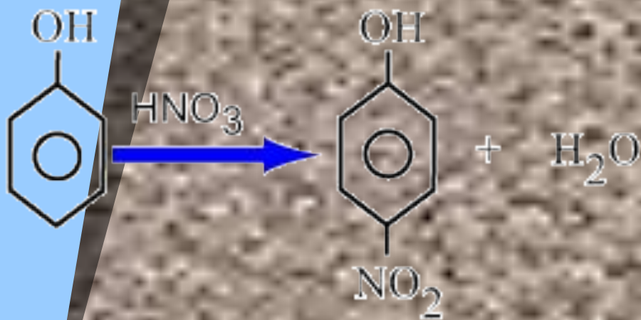
пара-нитрофенол
