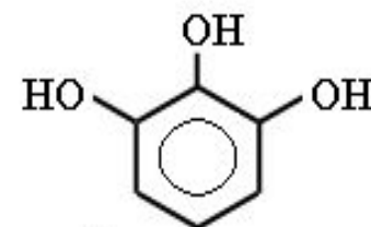
Пирогаллол (1,2,3-тригидроксибензол)
