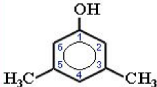
3,5-диметилфенол
