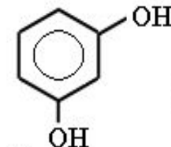
Резорцин (1,3-дигидрокси-бензол)
