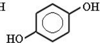
Гидрохинон (1,4-дигидрокси-бензол)
