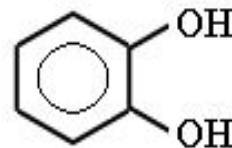
Пирокатехин (1,2-дигидрокси-бензол)
