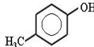
пара -Крезол (1-гидрокси-4-метилбензол)
