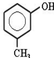
мета -Крезол (1-гидрокси-3-метилбензол)
