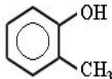
орто -Крезол (1-гидрокси-2-метилбензол)
