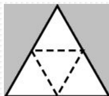
Тетраэдр
