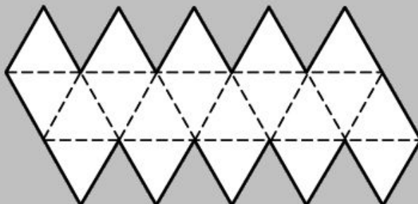
Икосаэдр
