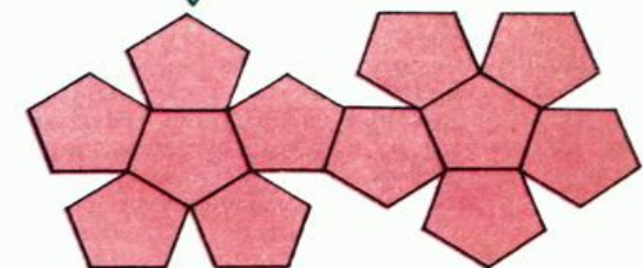
Додекаэдр
