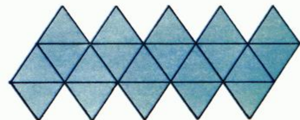
Икосаэдр
