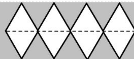
Октаэдр
