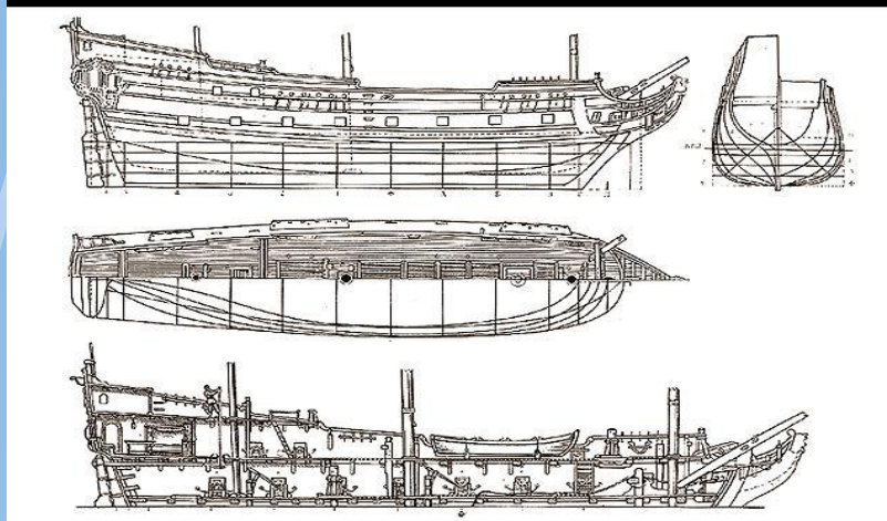
Теоретический чертеж и продольный разрез корабля "Орел" 1669 год
