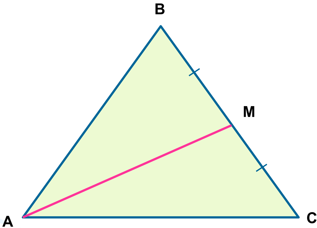
медіана трикутника
