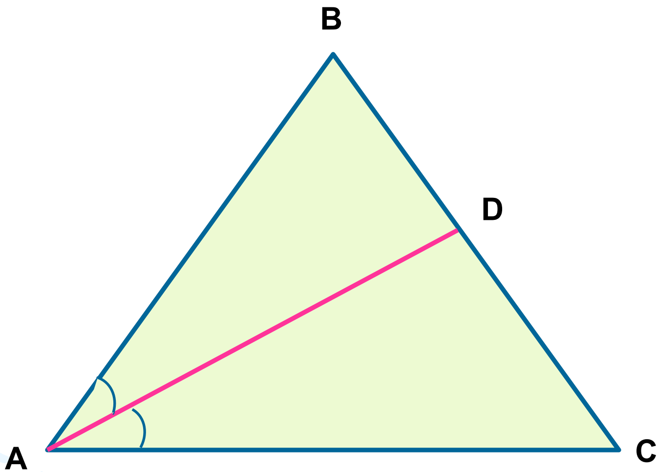
Биссектриса треугольника
