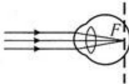
Близорукий глаз
