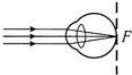
Нормальный глаз
