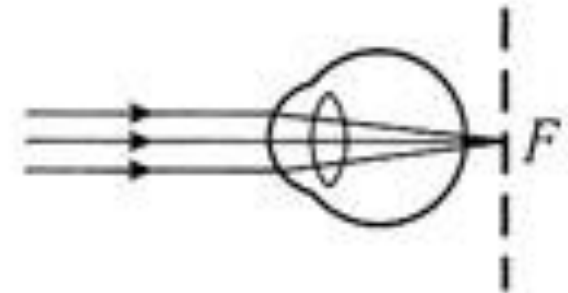
Дальнозоркий глаз
