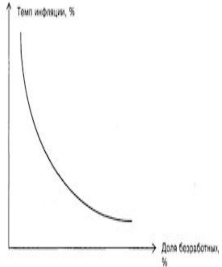
Рис. III.1. Кривая Филлипса
