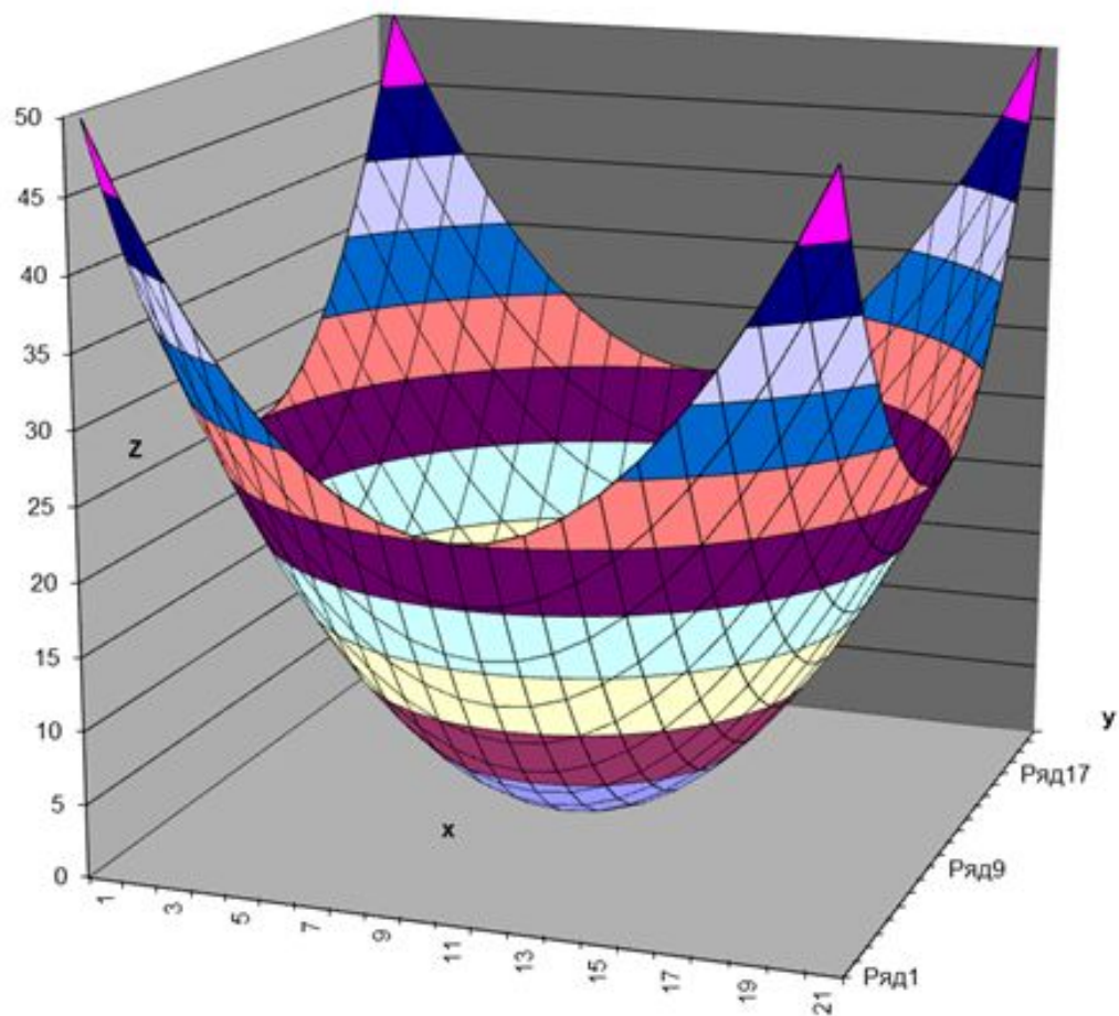
График эллиптического параболоида
