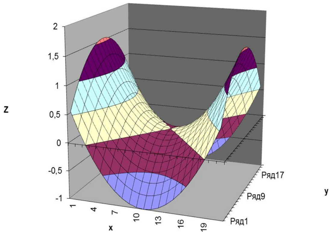
График гиперболического параболоида
