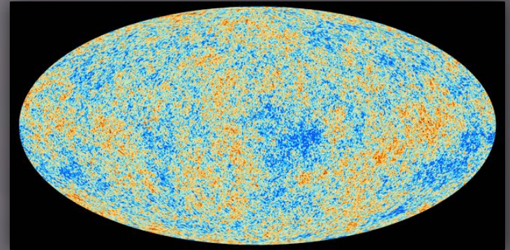
Реликтовое излучения.
