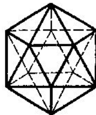
Икосаэдр
