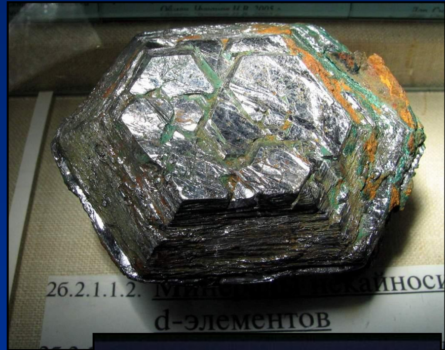
Молибденит \text{MoS}_2
