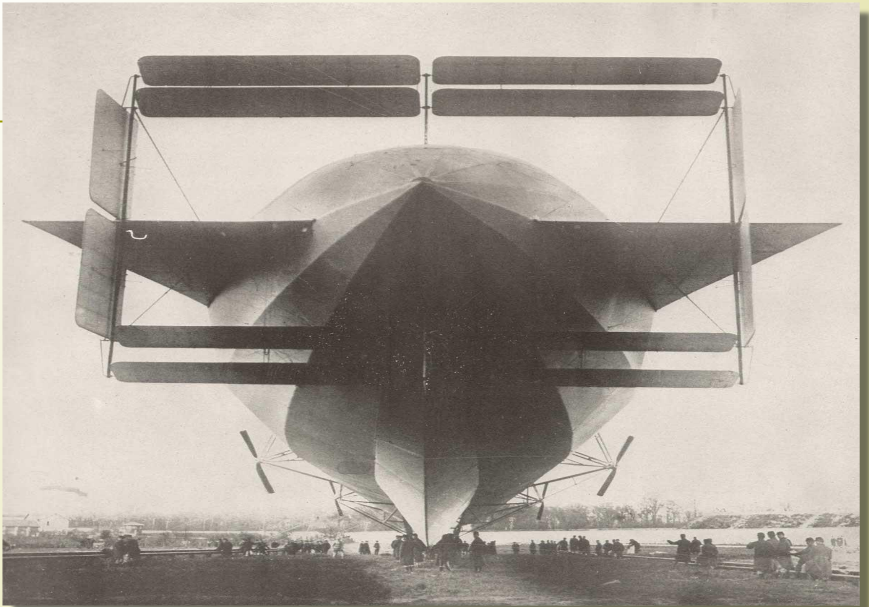
Французский дирижабль
