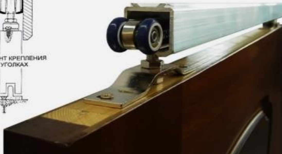
Рельс механизма с ограничителем
