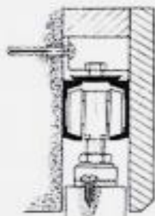
ВАРИАНТ КРЕПЛЕНИЯ НА УГОЛКАХ
