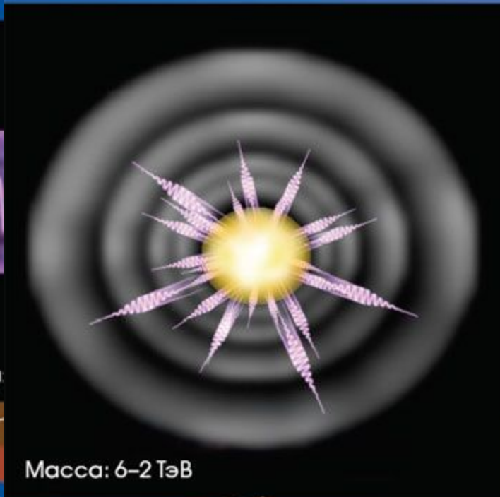
Шварцшильдовская стадия
