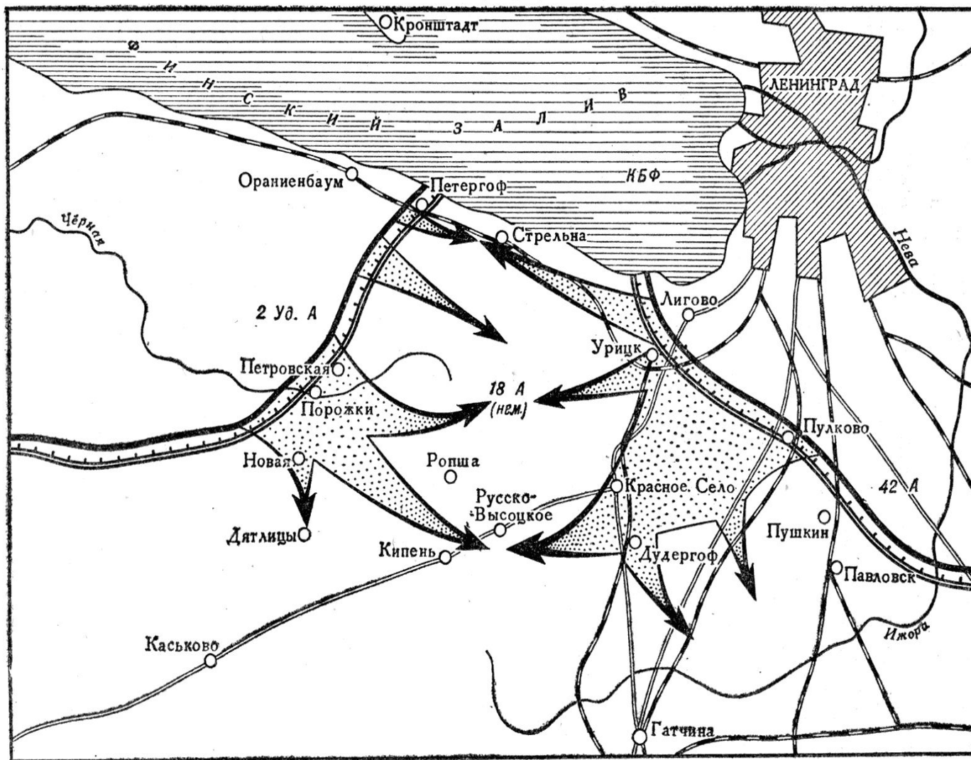
СХЕМА БОЕВ ЗА ПОЛНОЕ СНЯТИЕ БЛОКАДЫ ЛЕНИНГРАДА (14—27 января 1944 г.)
