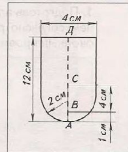
Рис. 118. Чертеж детали
