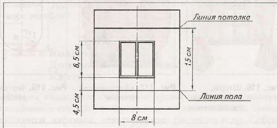
Рис. 115. Чертеж макета окна
