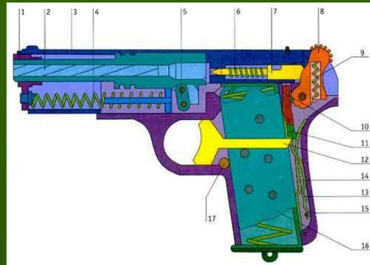
Схема пистолета ТТ
