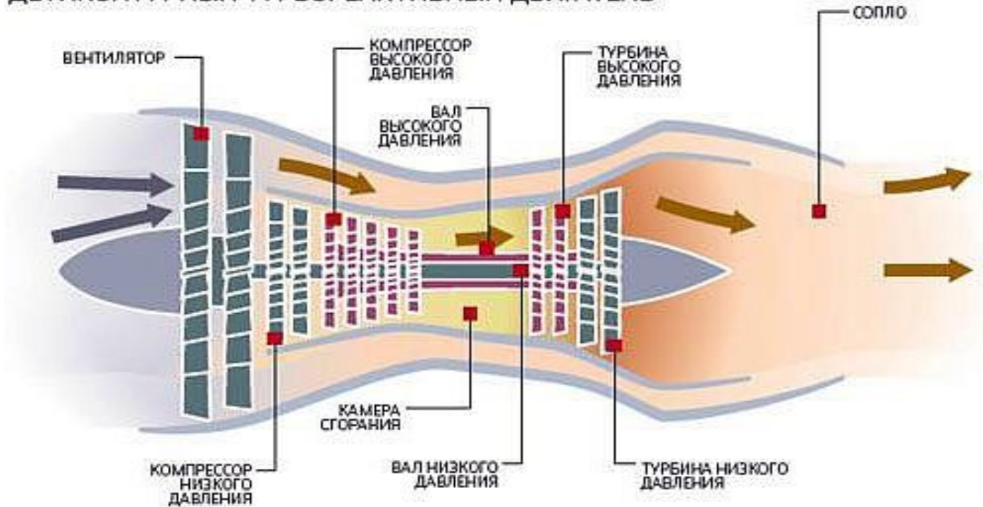
ДВУХКОНТУРНЫЙ ТУРБОРЕАКТИВНЫЙ ДВИГАТЕЛЬ
