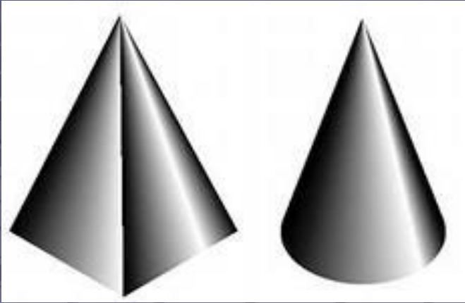
конус
