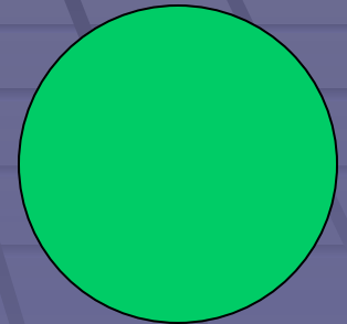
цилиндр
