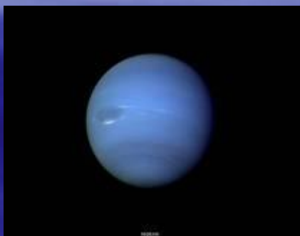
Нептун
