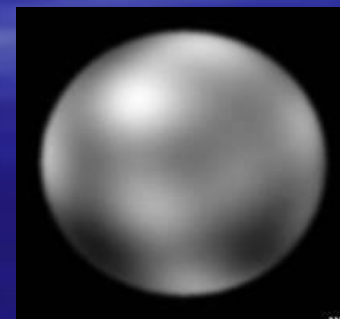
Плутон
