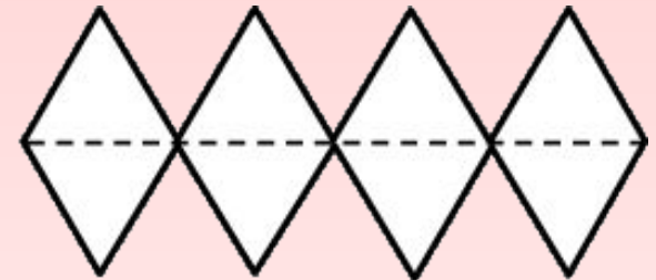
Октаэдр
