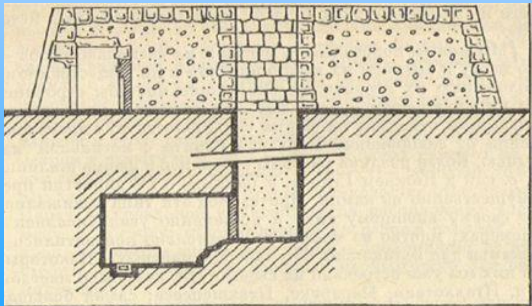
Разрез мастабы. Слева моелельня, посредине шахта, ведущая в подземную часть с камерой и саркофагом
