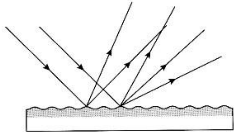
Диффузное (рассеянное)
