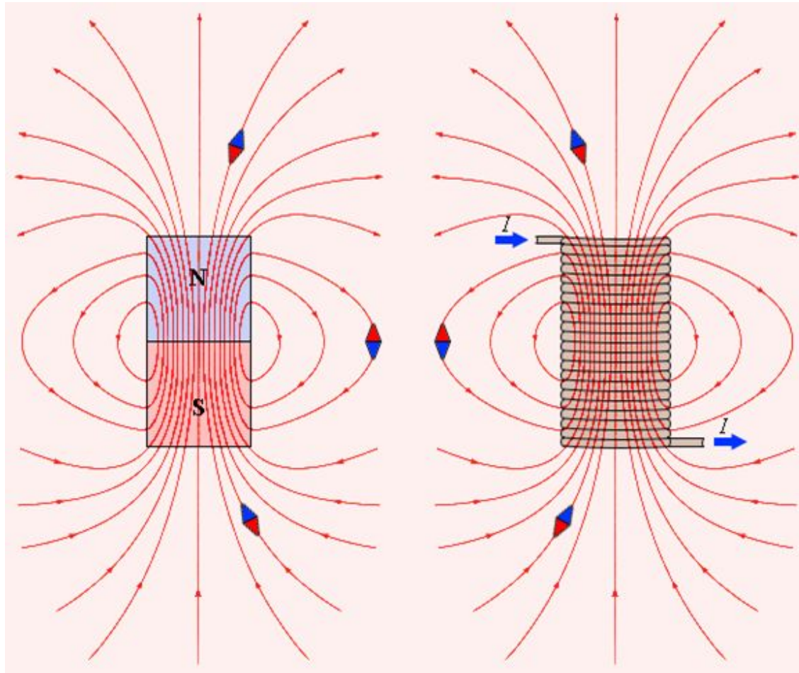
Магнитное поле постоянного магнита.
