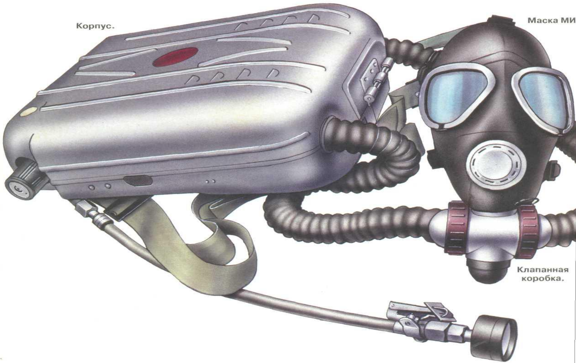
Кислородный изолирующий противогаз (КИП-8)
