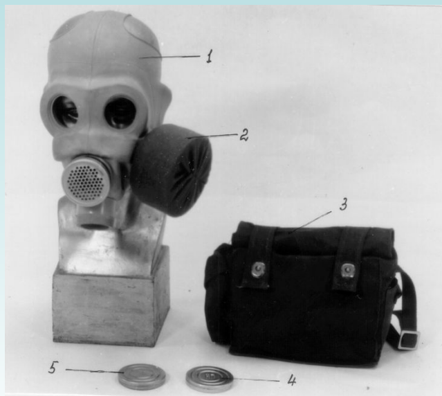
1 - шлем-маска ШМГ; 2 - фильтрующе-поглощающая коробка ЕО-18К в чехле; 3 - сумка; 4 - непотепляющие пленки; 5 - мембраны переговорного устройства
