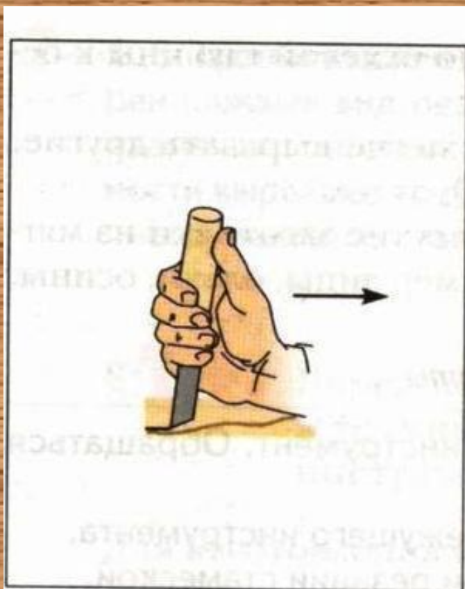
Рис. 51. Захват и положение инструмента при резьбе
