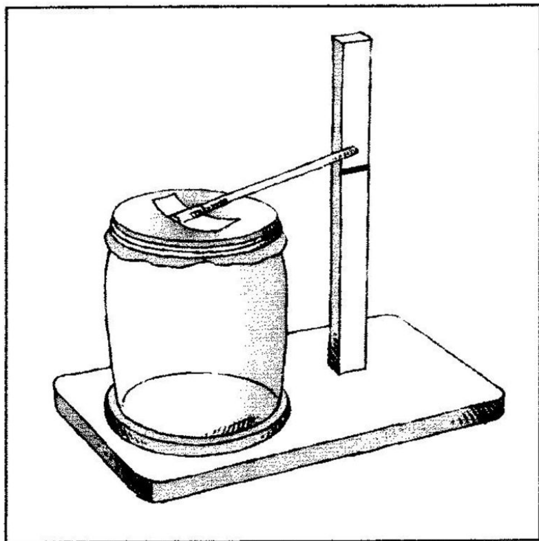
Резиновый барометр при высоком давлении.
