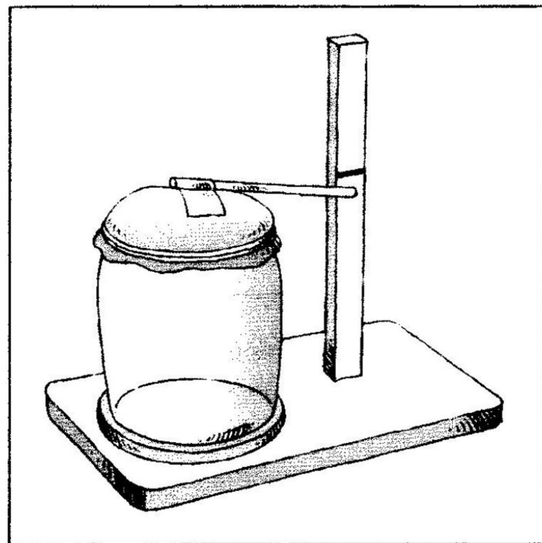
Резиновый барометр при низком давлении.
