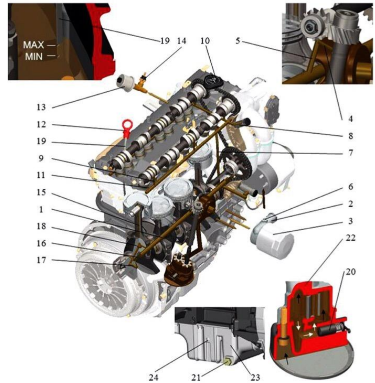
Схема системы смазки:
