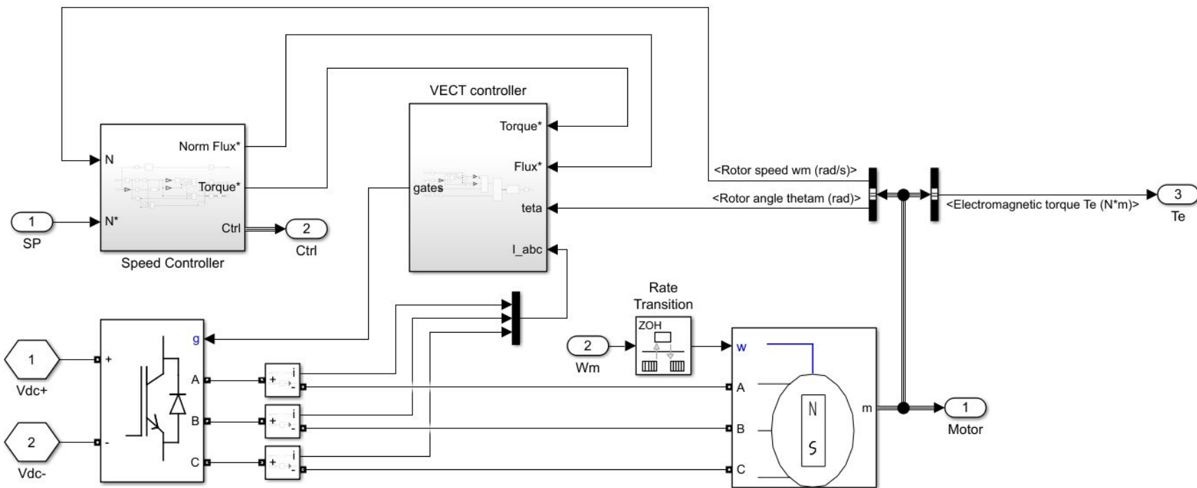
Схема блока PM Synchronous Motor Drive
