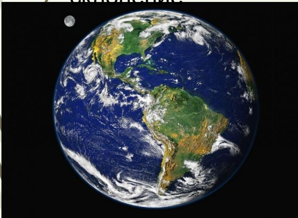
Земля-1 склонение
