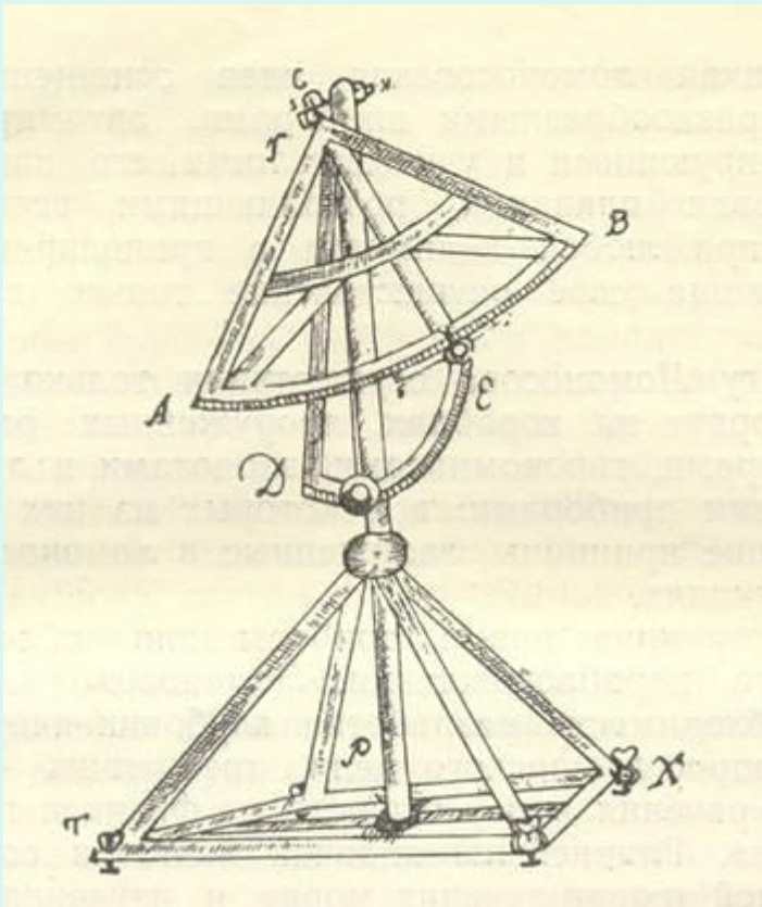
Прибор для определения полуденной линии. Рисунок М. В. Ломоносова.
