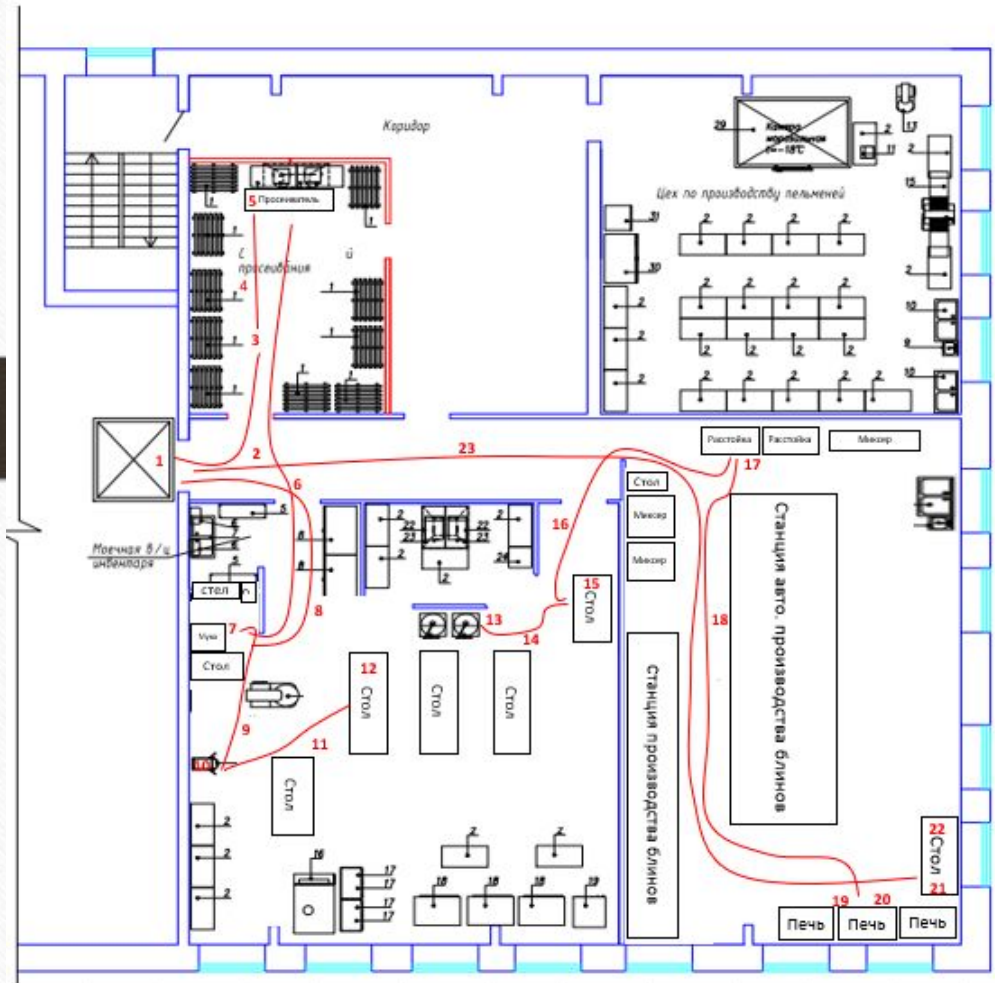
План четвертого этажа
