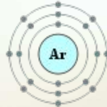
Схема атома аргона
