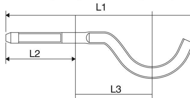
Вариант крепления с помощью анкера
