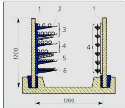
Схема прокладки кабелей в канале
