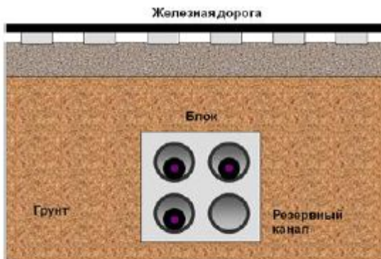
Схема прокладки кабелей в блоке
